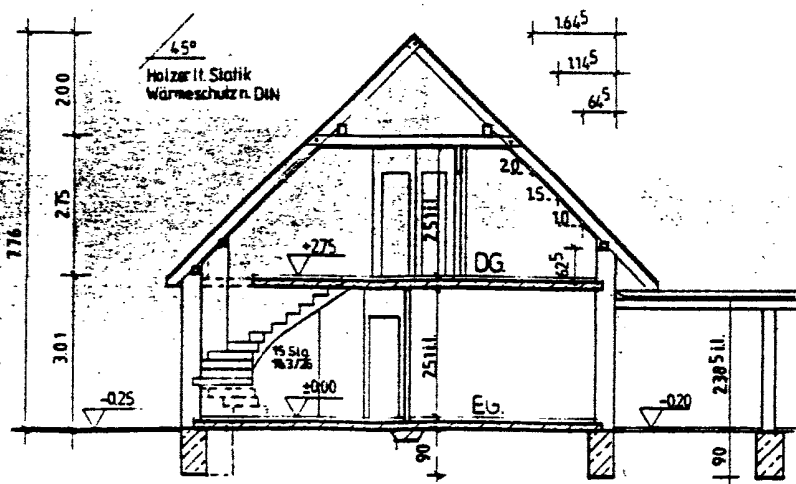
Schnitt A-B
