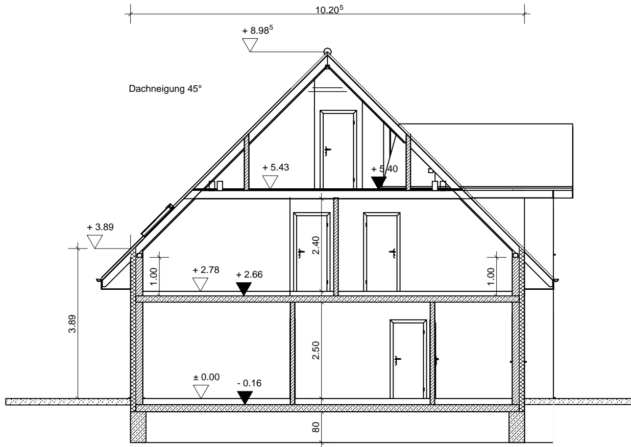
Schnitt Wohnhaus
